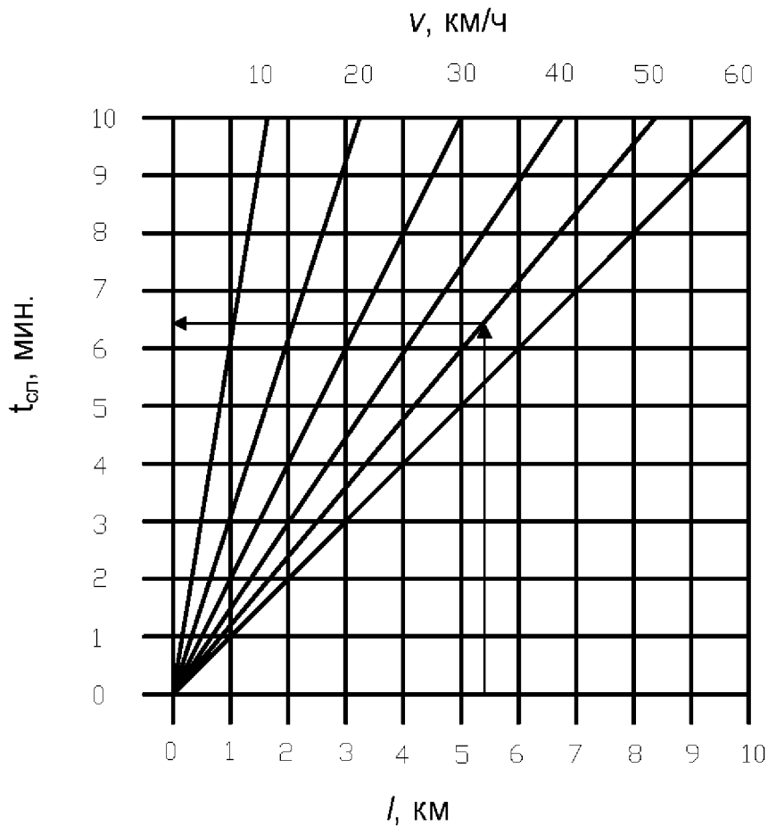
Рисунок Б.1 - Номограмма для определения времени следования подразделения пожарной охраны к месту вызова
