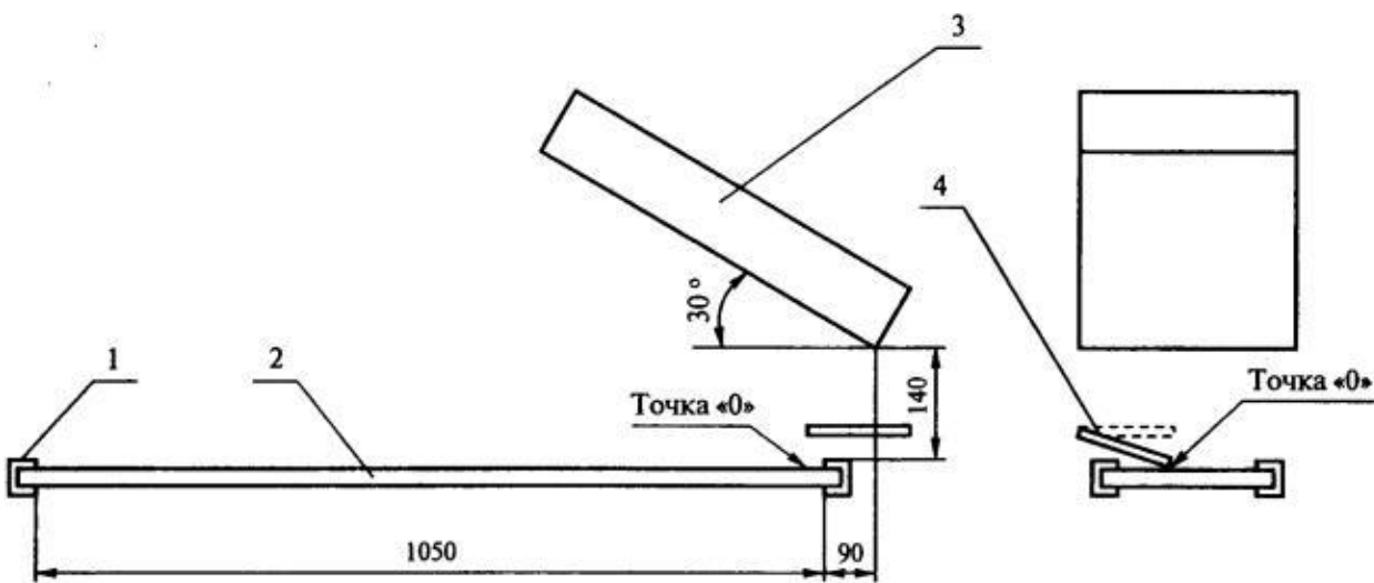
Рисунок 2 -Схема взаимного расположения радиационной панели, образца и газовой горелки
