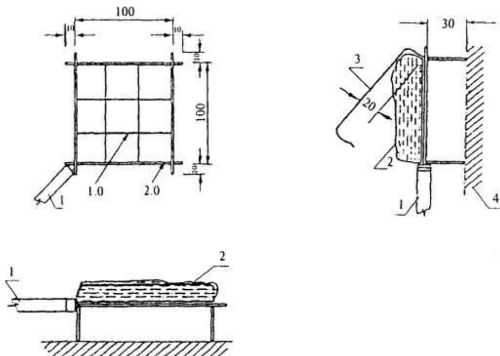
Рисунок Б.1 - Рамка для закрепления ватного тампона
