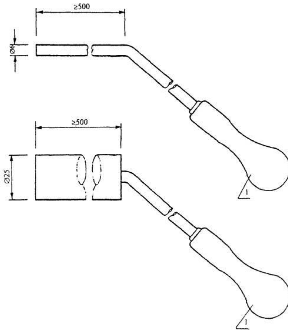
Рисунок Б.2 - Конструкция щупов
