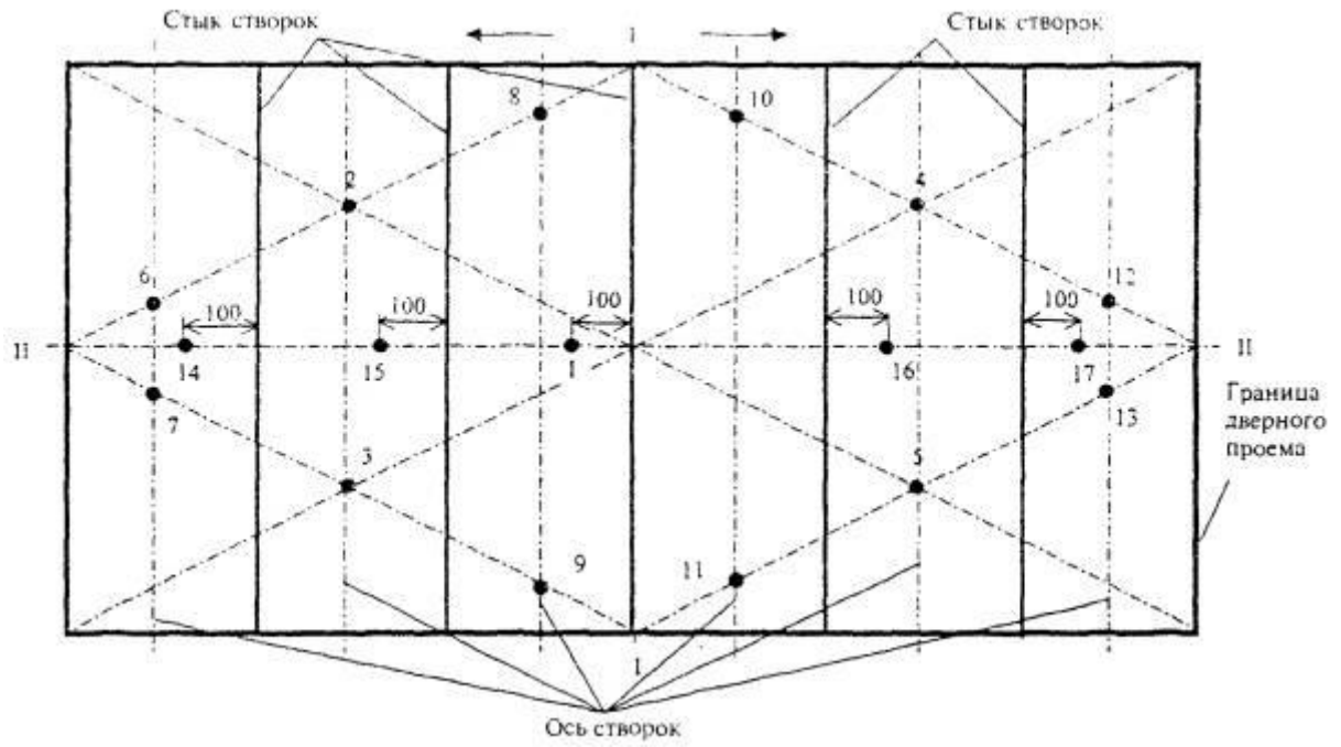
Рисунок А.5 - Схема установки термопар на необогреваемой поверхности шестистворчатой горизонтально-раздвижной двери центрального открывания
