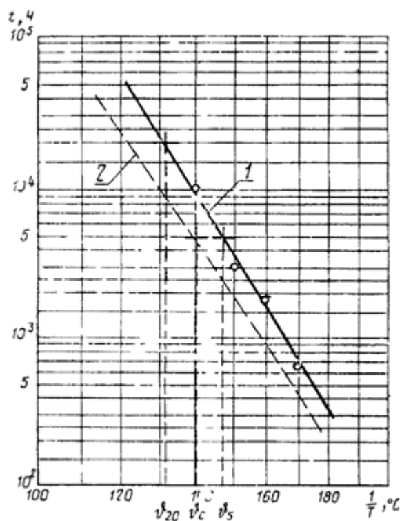
График срока службы эмаль-провода
