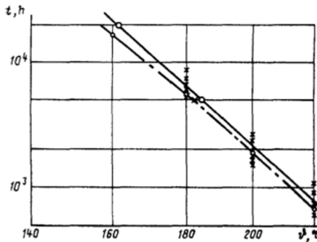
График сроков службы
