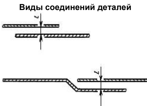
Черт.2. Виды соединений деталей
