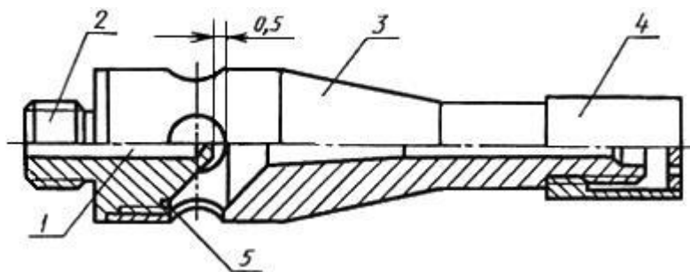
Черт.11. Конструкция газовой горелки
