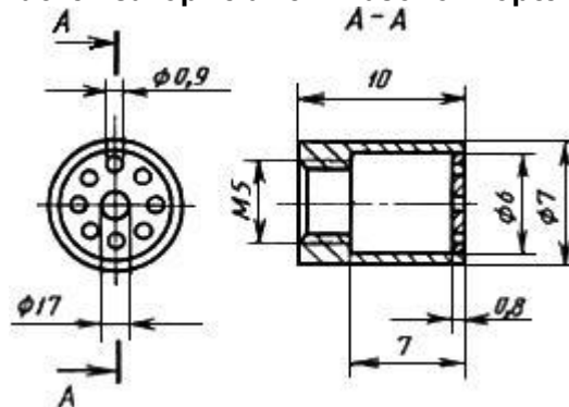
Стабилизатор пламени газовой горелки
