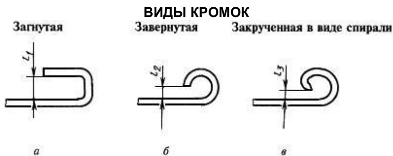
Черт.1. Виды кромок
