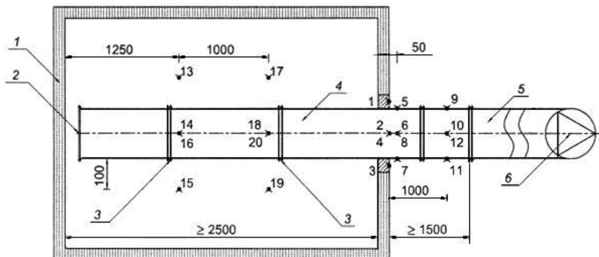
1 - печь; 2 - заглушенный торец образца; 3 - места сочленения элементов образца; 4 - испытываемый образец воздуховода (с отверстием или без него); 5 - переходной элемент; 6 - вентилятор; - ТЭП, установленные: 1-4 - на поверхности уплотнений воздуховода в проеме печи; 5-12 - на необогреваемых поверхностях воздуховода; 13-20 - в печи
