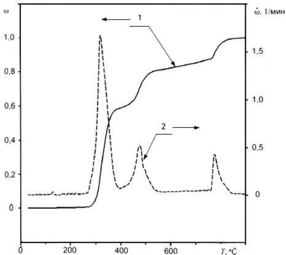
Рисунок А.2.1 - Характерные термоаналитические кривые образца материала
