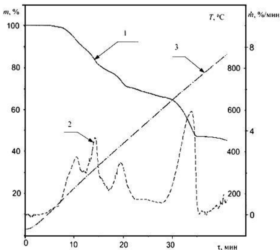
Рисунок А.1.1 - Характерные термоаналитические кривые образца материала
