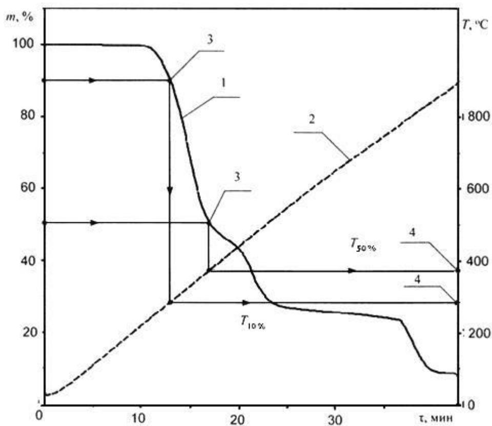
Рисунок В.1 - Схема определения характерных значений температуры при фиксированных значениях потери массы (в координатах "потеря массы - время")
