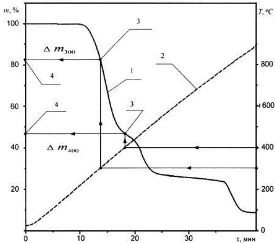
1 - ТГ-кривая (потеря массы); 2 - температура; 3 - характерные точки ТГ-кривой; 4 - потеря массы при 300 °С и 400 °С
