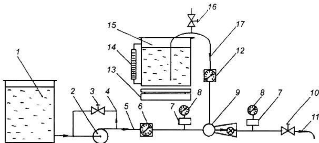
Рисунок 2 - Установка для определения расхода воды и пенообразователя через дозатор
