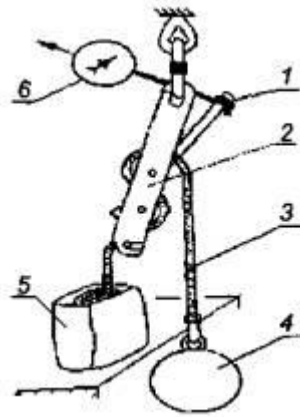
Рисунок 1 - Схема проверки величины тормозного усилия УКСПр
