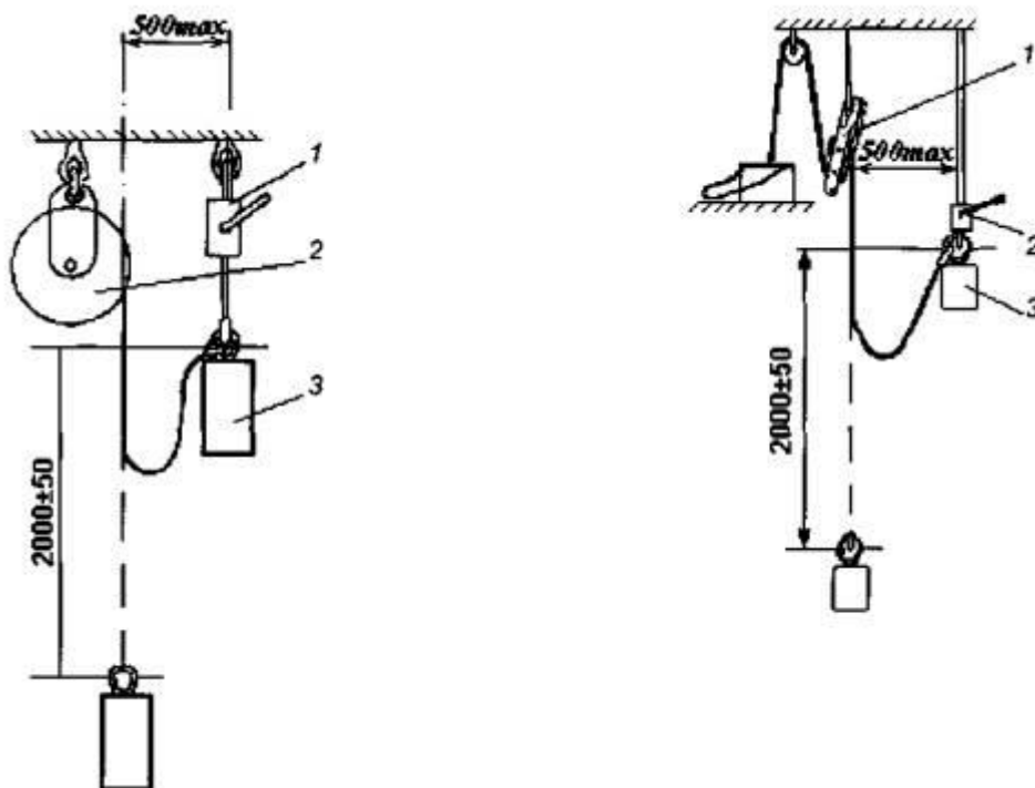
схема испытания УКСПа
