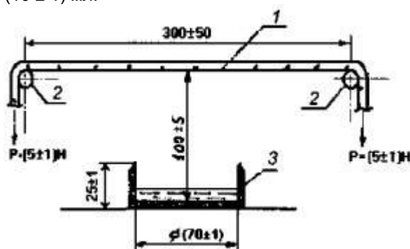
Рисунок 6 - Схема испытаний образца каната (ленты) на воздействие открытого пламени
