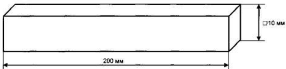
Рисунок А.1 - Стержень для проведения испытания по 8.11
