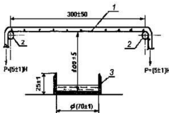
1 - образец веревки; 2 - опоры; 3 - емкость для горючего
