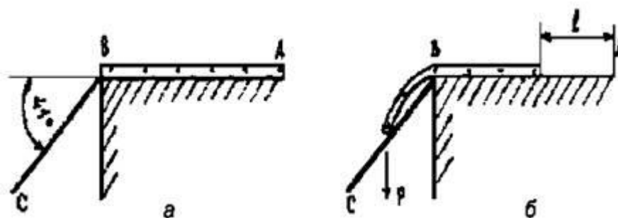
Рисунок 2 - Схемы испытаний по определению показателя жесткости образца веревки
