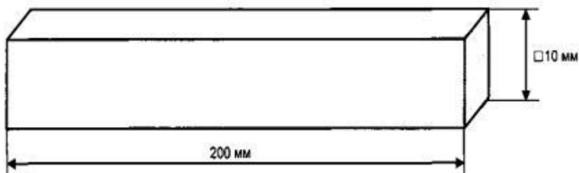
Рисунок А.1 - Стержень для проведения испытания по 8.11
