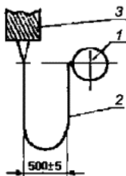
Рисунок 4 - Схема испытаний образца веревки на воздействие динамической нагрузкой
