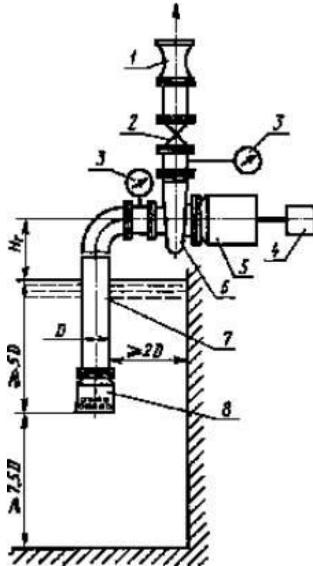
1 - устройство для измерения подачи; 2 - напорная задвижка; 3 - прибор для измерения давления; 4 - тахометр; 5 - приводной двигатель мотопомпы; 6 - насос мотопомпы; 7 - всасывающая линия; 8 - всасывающая сетка
