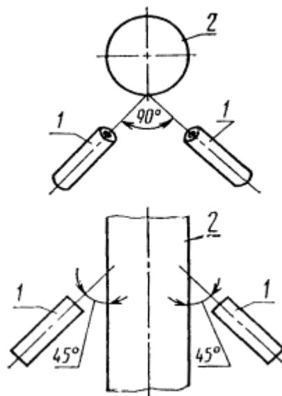
1 - горелка; 2 - образец
