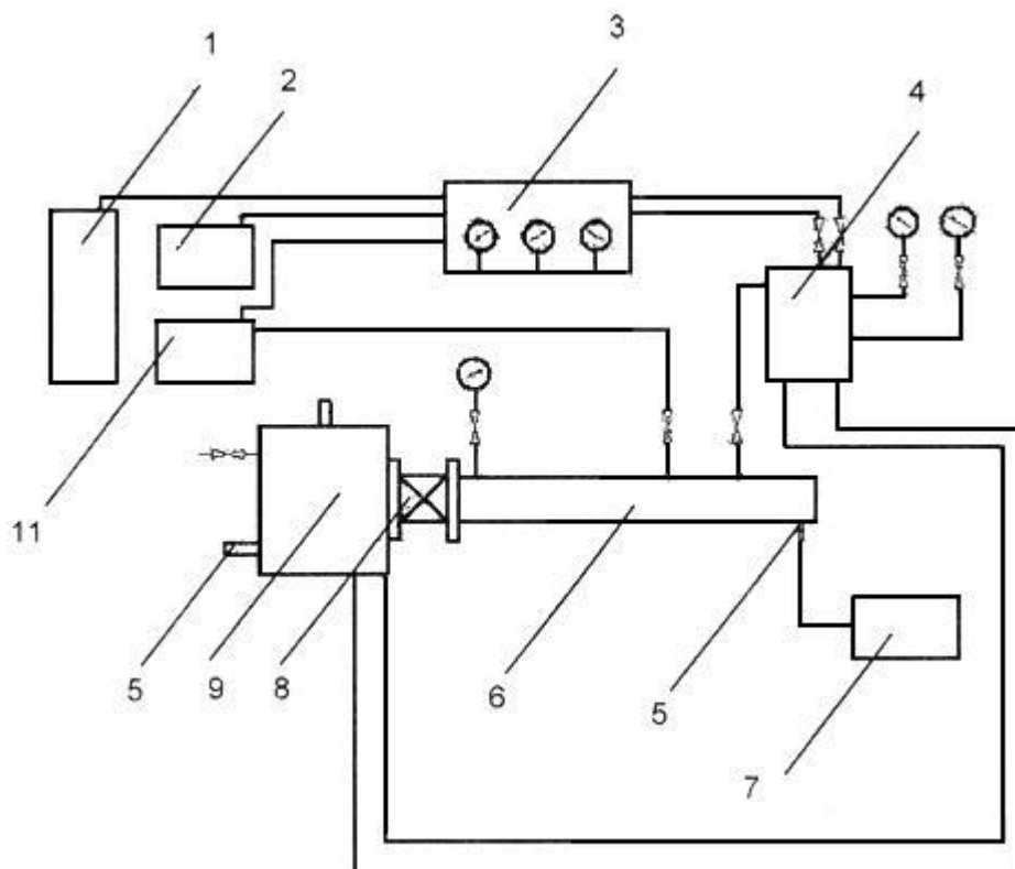
Рисунок 1 - Принципиальная схема экспериментального стенда
