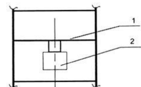
Рисунок 2 - Испытание ступеньки лестницы на величину остаточной деформации
