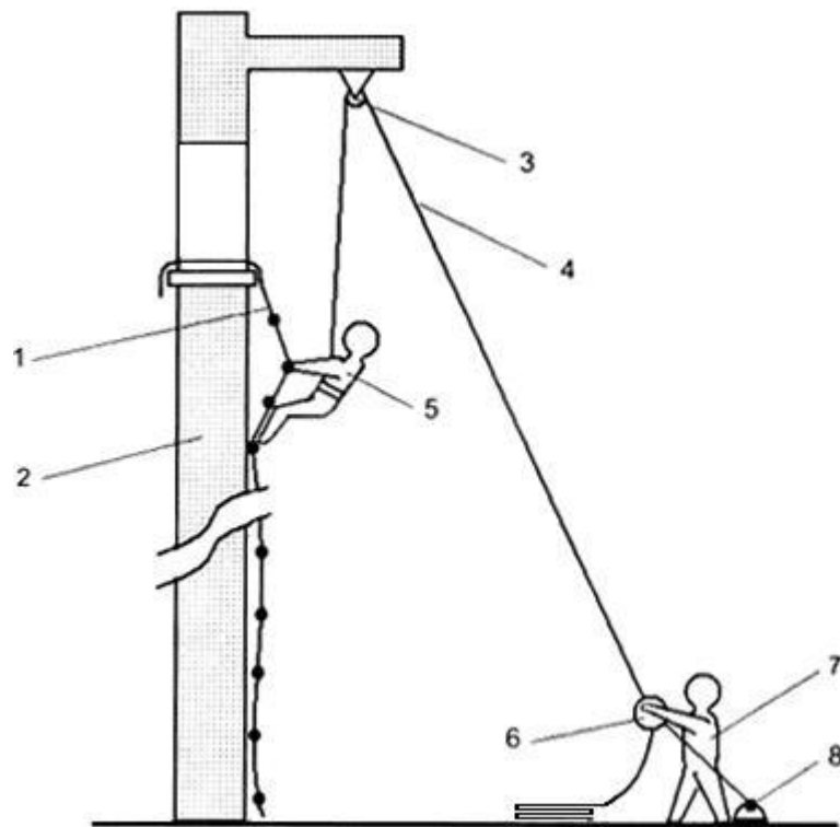
1 - лестница; 2 - здание; 3 - блок; 4 - страховочная веревка; 5 - испыталель; 6 - приспособление для экстренного торможения веревки; 7 - оператор, осуществляющий страховку испыталелья; 8 - якорь
