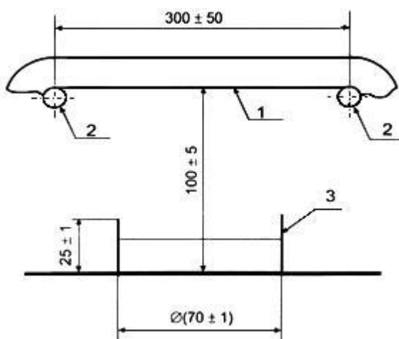
Рисунок 5 - Схема испытаний образца ступеньки и тетивы лестницы на воздействие открытого пламени
