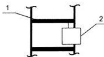
Рисунок 3 - Испытание ступеньки лестницы на срез
