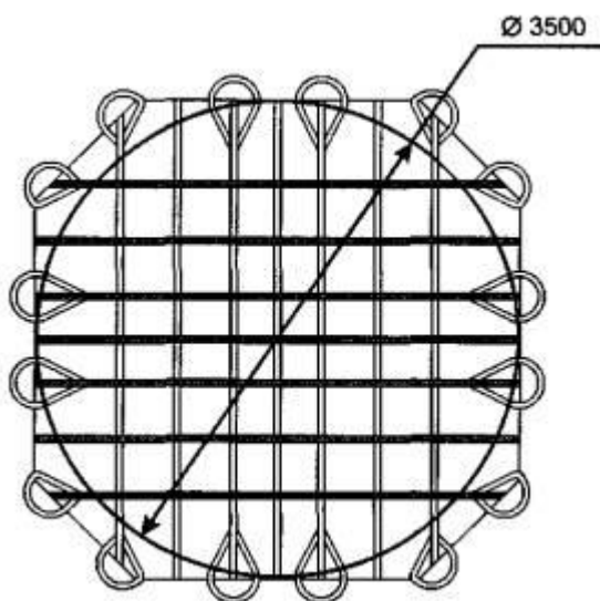
Рисунок 1 - Конструкция ПСН
