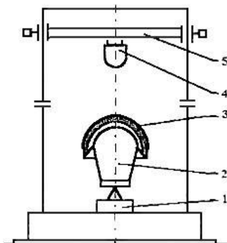
Рисунок 1 - Принципиальная схема стенда
