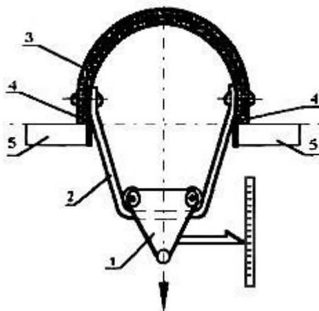
Рисунок 2 - Принципиальная схема устройства для проверки прочности подбородочного ремня
