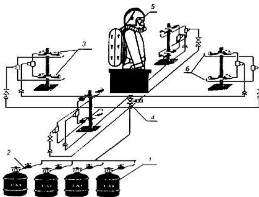
Рисунок Б.1 - Схема стенда "Термоманекен"
