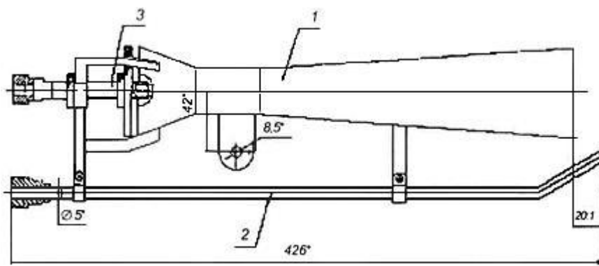
Рисунок Б.2 - Схема горелки
