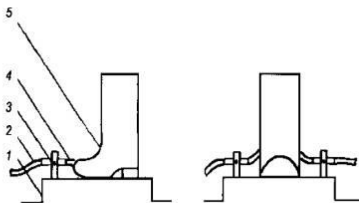
Рисунок 2 - Схема установки
