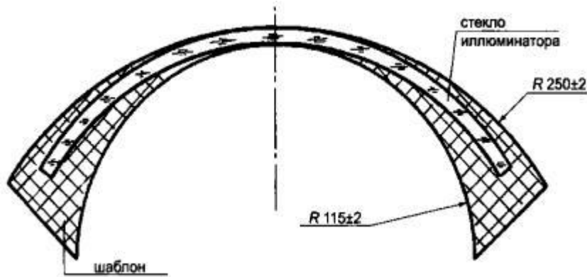
Рисунок 10 - Определение радиуса изгиба стекла иллюминатора
