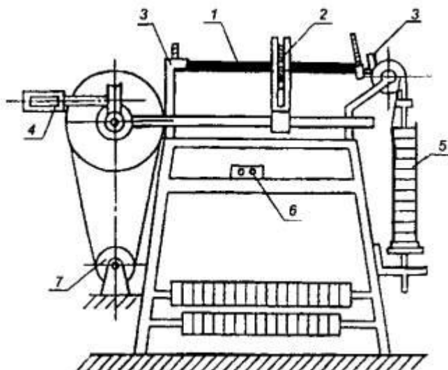
Рисунок 3 - Установка для определения устойчивости материалов к истиранию
