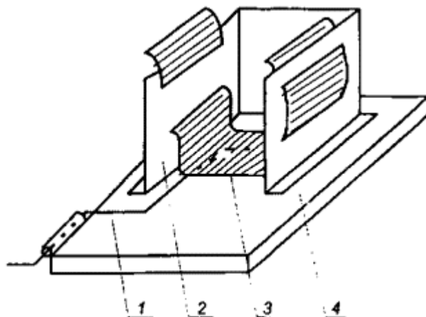
1 - термоэлектрический преобразователь; 2 - держатель; 3 - исследуемый образец; 4 - керамическая пластина
