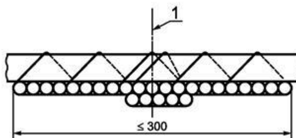
1 - центральная линия лестницы
