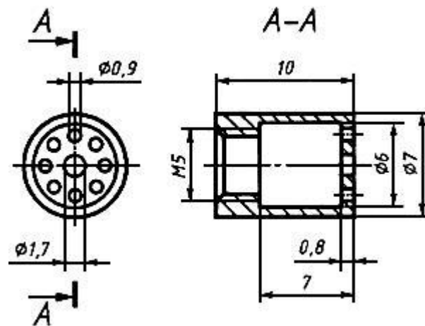
Рисунок А.4 - Схема стабилизатора пламени
