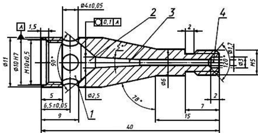
1 - воздушная камера; 2 - зона смешивания газа; 3 - зона диффузии; 4 - выпускное отверстие
