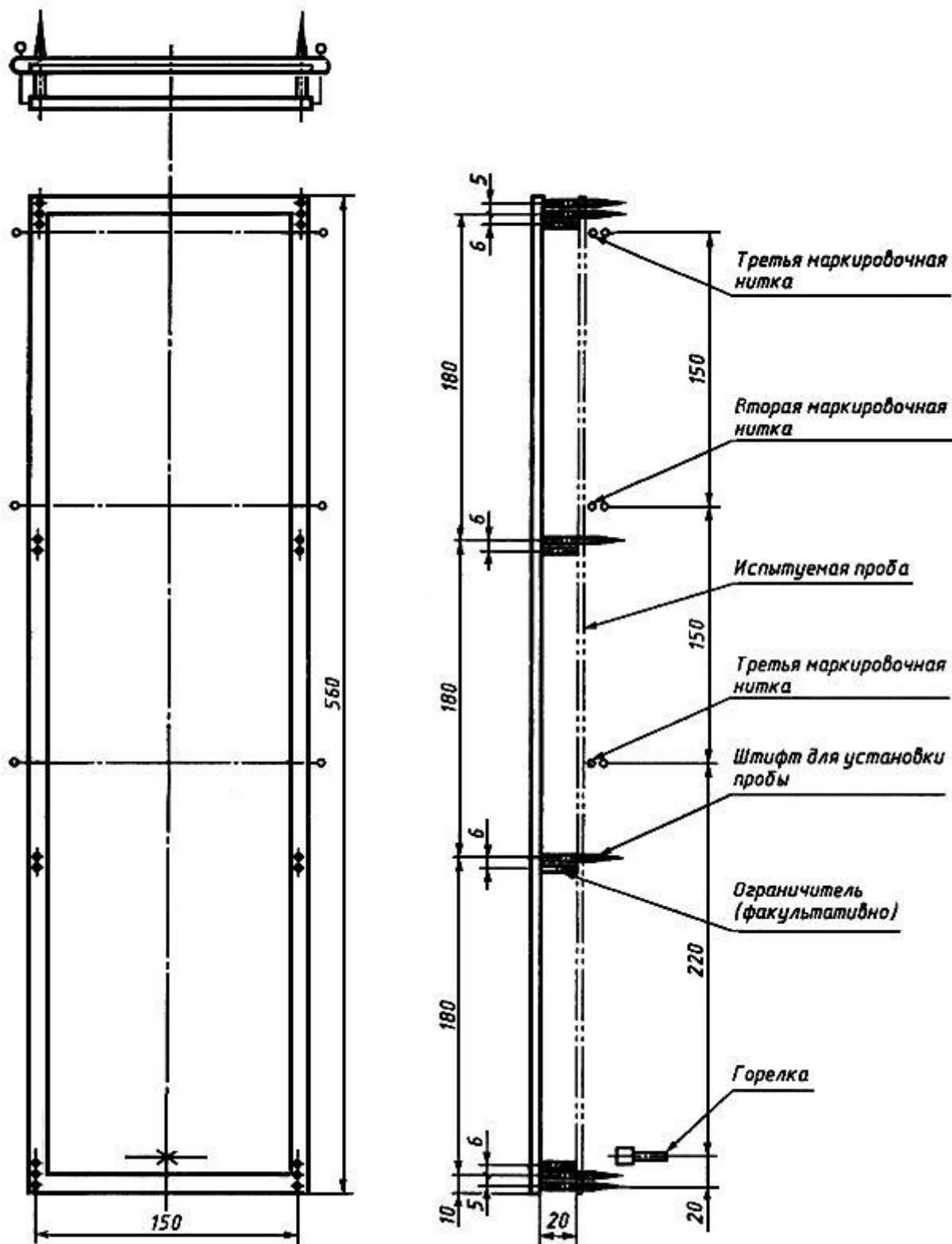
Рисунок 1 - Схема держателя для элементарной пробы
