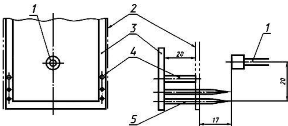
Рисунок 2а - Размещение горелки при поверхностном зажигании
