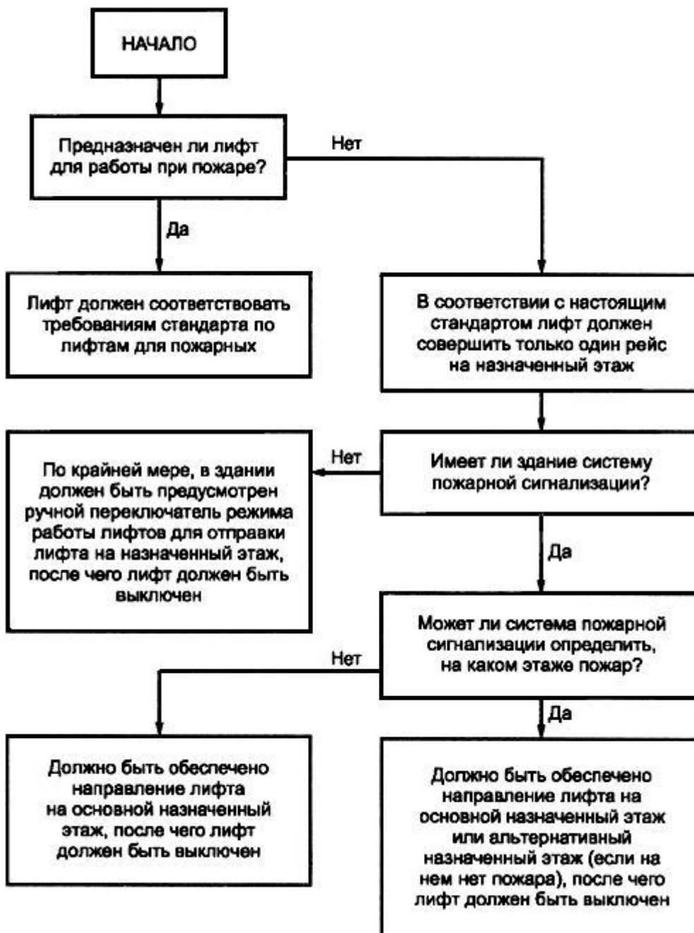
Рисунок А.1. Блок-схема формирования требований к лифту при пожаре
