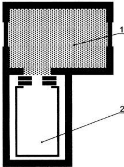
Рисунок В.1 - Схема (план) размещения одиночного лифта для пожарных и пожарозащищенного лифтового холла
