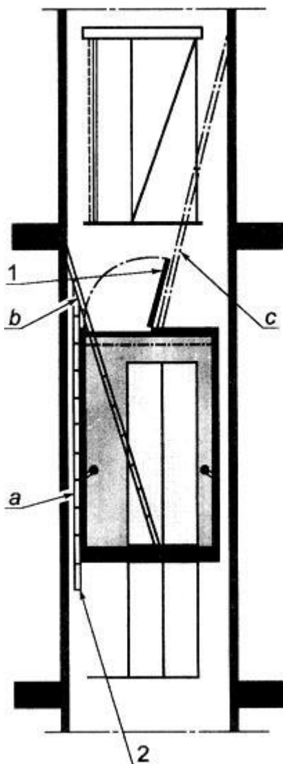
Рисунок G.1 - Схема высвобождения людей из застрявшей кабины с использованием передвижной лестницы, закрепленной снаружи кабины
