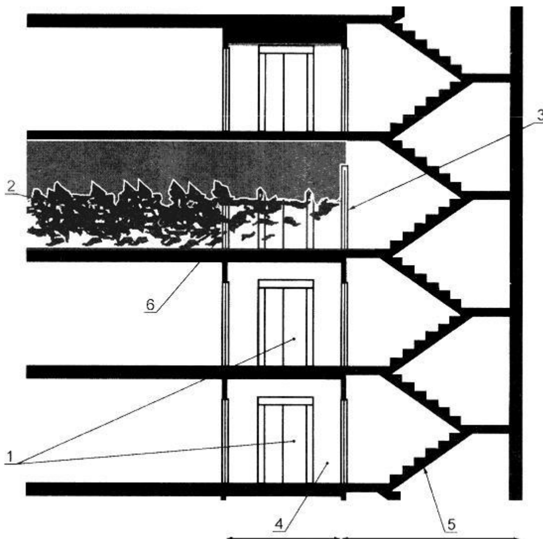
Рисунок А.2 - Случай проникновения огня в пожарозащищенный лифтовой холл
