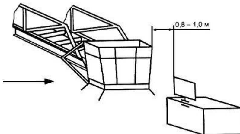
Рисунок Б.4 - Движение вершины лестницы с люлькой при повороте подъемно-поворотного основания
