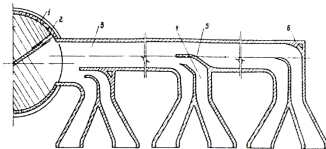
Рис. 7. Газопроводы с улучшенной аэродинамической характеристикой:
