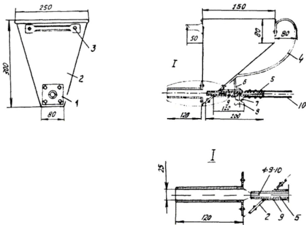
Рис. 9. Ручной бетономет:
