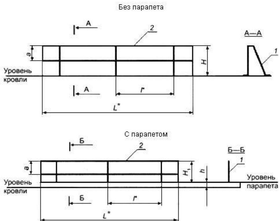
Рисунок Г.1 - Ограждения кровли
