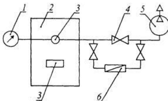
1 - микроманометр; 2 - камин; 3 - манжета резиновая; 4 - кран проходной; 5 - вакуум-насос; 6 - расходомер
