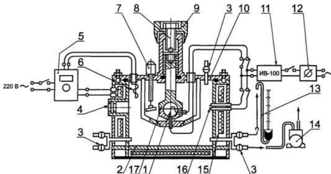
Рисунок 1 - Установка для определения БЭМЗ
