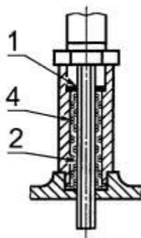
б) Трубный ввод
