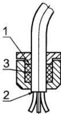
б) Трубный ввод
