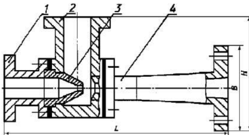
1 - входной патрубок; 2 - всасывающая камера; 3 – сопло; 4 - выходной патрубок
