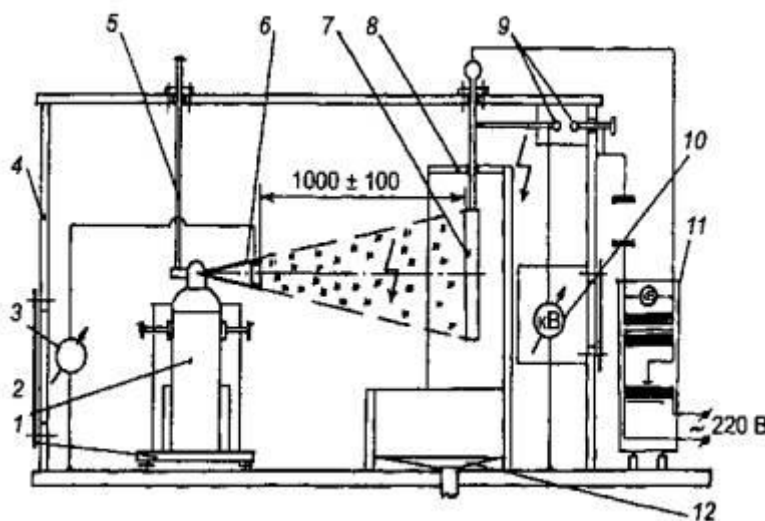
1 - изолирующая подставка; 2 - испытуемый огнетушитель; 3 - измеритель тока утечки; 4 - защитный каркас испытательного стенда; 5 - устройство дистанционного запуска огнетушителя; 6 - насадка огнетушителя с электропроводящим элементом; 7 - мишень; 8 - экран; 9 - разрядник; 10 - киловольтметр; 11 - источник высокого напряжения; 12 - емкость для сбора отработанного ОТВ
