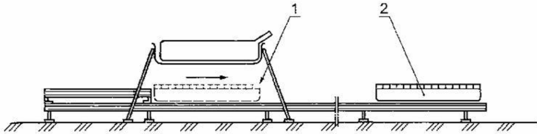
1 — решетка; 2 — металлический поддон Рисунок 4 — Фаза D. Окончание испытания
