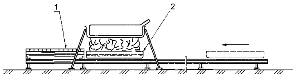
Рисунок 2 — Фаза В. Свободный контакт с пламенем
