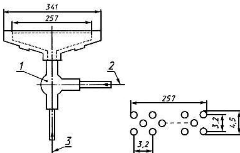
Рисунок 4 - Горелка
