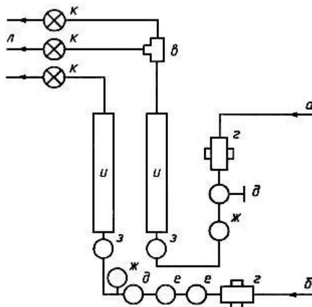
Рисунок 5 - Типовая система контроля расхода газа
