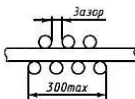
Рисунок 3в - Несоприкасающиеся кабели, закрепленные на общих сторонах стандартной лестницы (A (F/R) > 35 мм )
