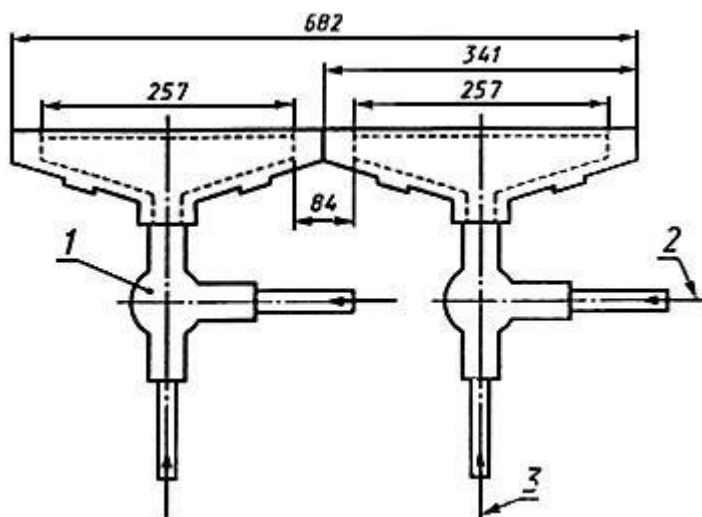
Рисунок 4а - Сдвоенная горелка
