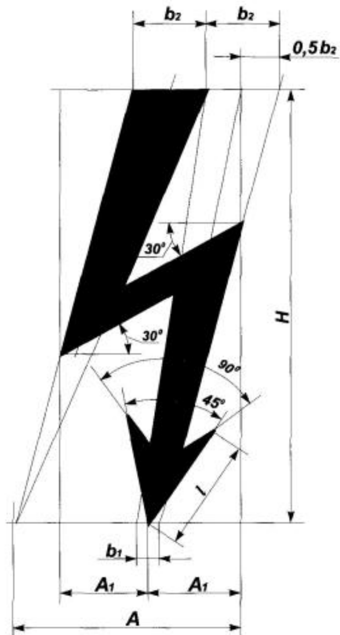
Рисунок Л.1 - Графический символ электрического напряжения
